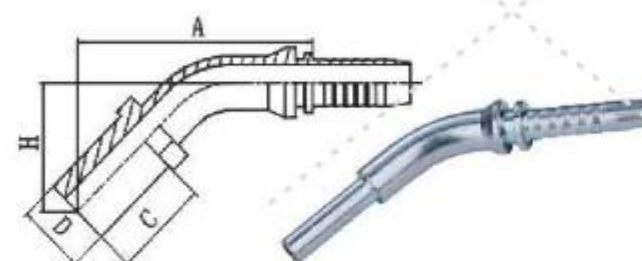
50041 45° 公制DIN2353卡套式直管 45° METRIC STANDPIPE STRAIGHT DIN 2353
