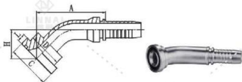
87341 45° SAE 法兰3000 PSI 45° SAE FLANGE 3000 PSI ISO12151-3-SAE J516
