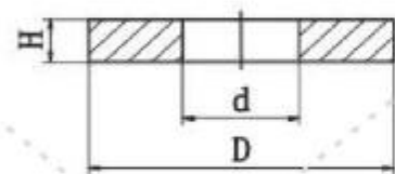
压力表紫铜垫片 Gauge copper gasket
