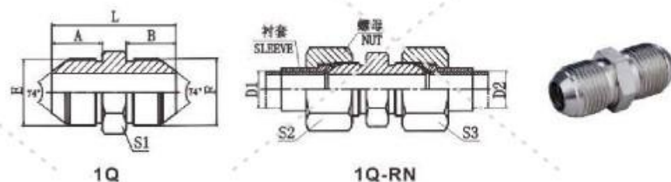
公制外螺纹74° 外锥 METRIC MALE 74° CONE
